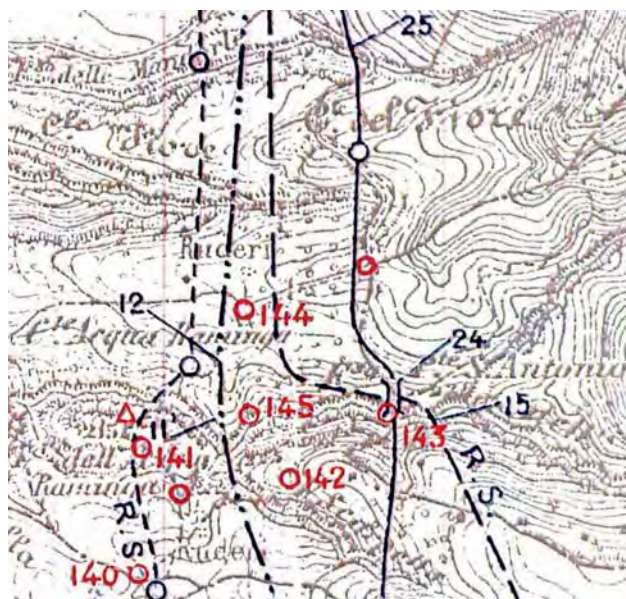
Fig. 1 – Il percorso dei quattro acquedotti Anienesi nel tratto che discende verso il Fosso dell'Acqua Raminga, con indicazione di capisaldi e livellazioni nella pianta tracciata da Ashby (1935).
