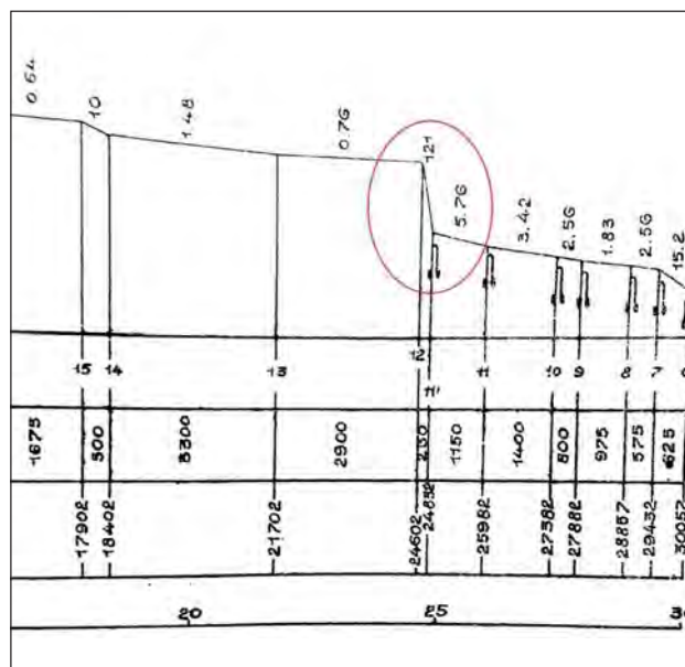
Fig. 2 – Particolare della curva di livellazione dell'acquedotto Marcia disegnata dal Reina (1917).
