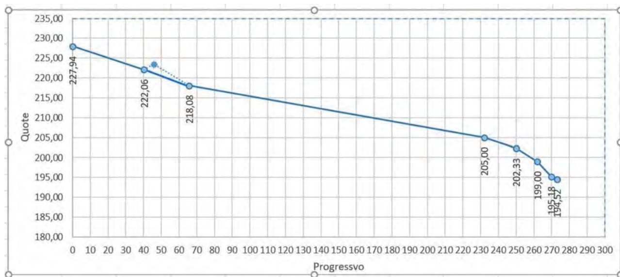
Fig. 23 – Profilo altimetrico dell'acquedotto.
