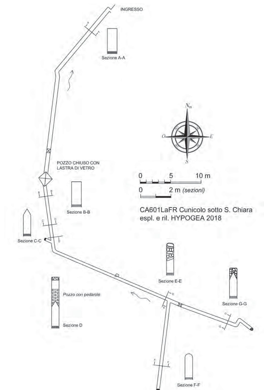
Fig. 12 – Rilievo topografico cunicolo di S. Chiara (©Hypogea). Fig. 12 – Location map of the conduct under S. Chiara (©Hypogea).
