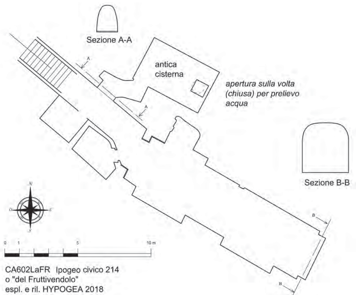
Fig. 30 – Rilievo topografico ipogeo sotto al negozio di Corso Vittorio Emanuele 214 (©Hypogea).
