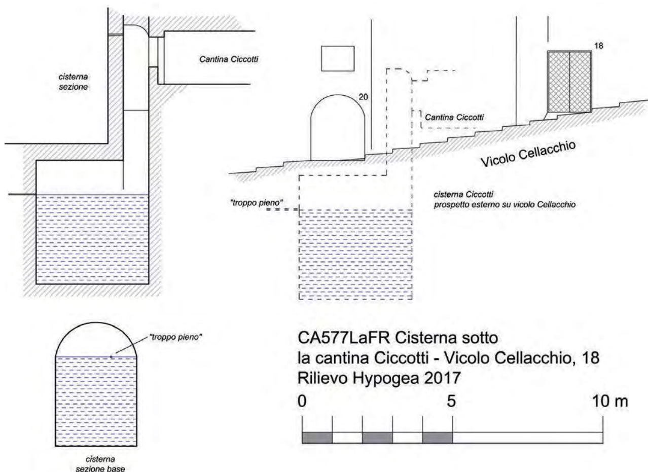
Fig. 9 – Rilievo topografico pozzo cisterna di Vicolo del Cellacchio (©Hypogea).
