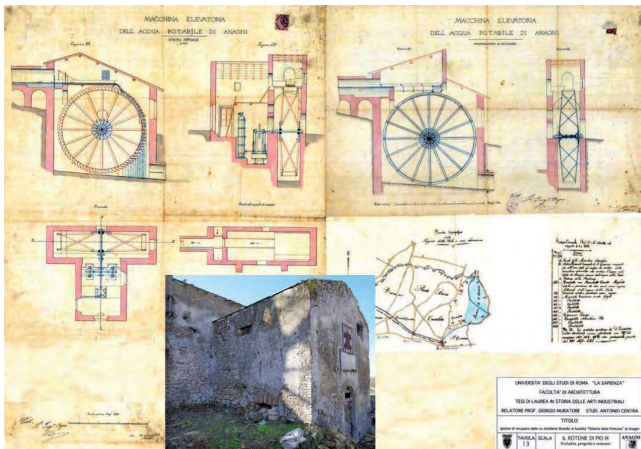
Fig. 11 – Progetto della macchina elevatoria (da Centra, 2001) e in sovrapposizione edificio del Rotone (foto C. Germani).
