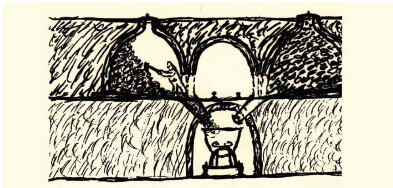
Fig. 11 – Schema di Funzionamento dei Forni Gill: il materiale estratto dalla miniera veniva caricato dall'alto nei forni dove attraverso il passaggio dei fumi da combustione lo zolfo si scioglieva e veniva convogliato in appositi contenitori. Una volta terminata l'estrazione il materiale di risulta veniva scaricato nelle gallerie sottostanti per essere trasportato all'esterno. (tratta dal Volume "Zolfo e Minatori nella Provincia di Pesaro e Urbino" di Giorgio Pedrocco - Arti Grafiche Stibu - Urbania - 2002).
