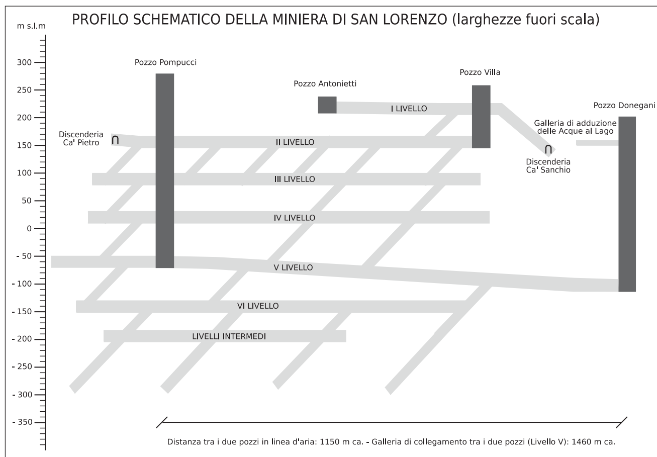
Fig. 2 - Schema esemplificato della sezione della miniera (disegno E.M. Sacchi).
