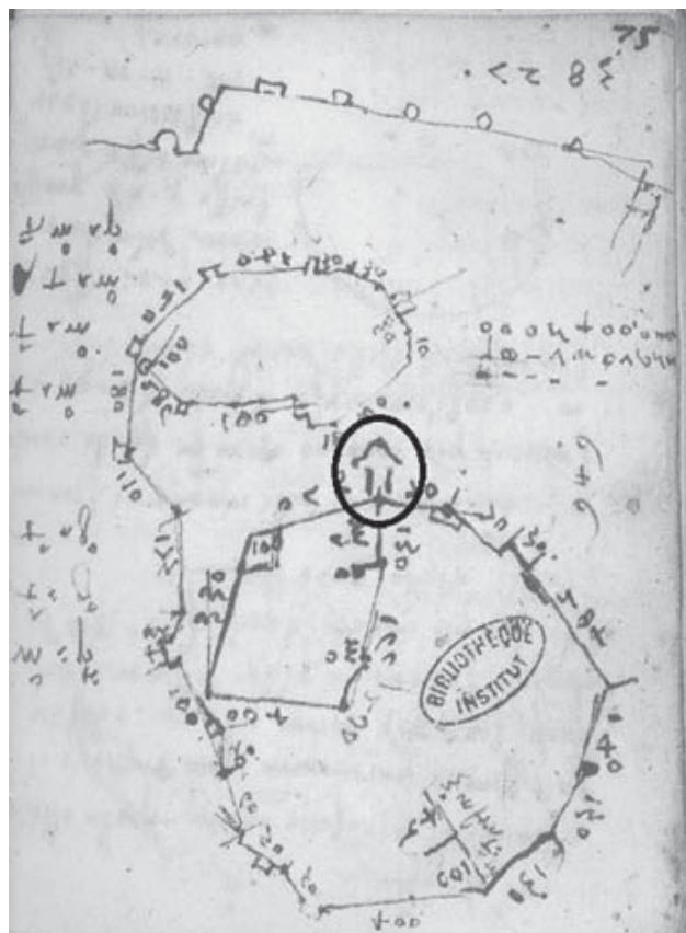
Fig. 4 - Ubicazione del torrione (nel cerchio) riportata da Leonardo da Vinci, Codice L, fol. 75 recto (1502). Adattato [M. Betti] da Nando De Toni, 1965, G. Barbera Editore.
