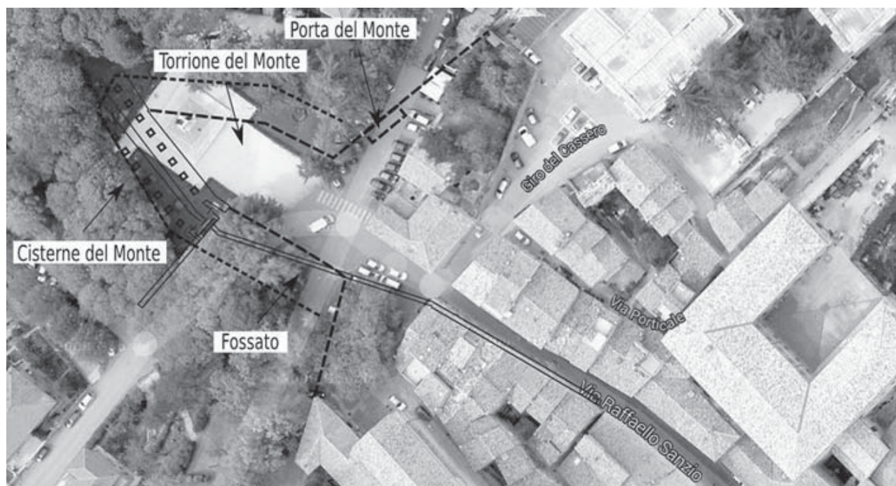
Fig. 8 - Ricostruzione della disposizione del torrione con la porta e le mura ora interrato, il fossato, i cunicoli di accesso e le cisterne su un'immagine satellitare dell'area del Belvedere del Monte (grafica: M. Betti & E.M. Sacchi).
