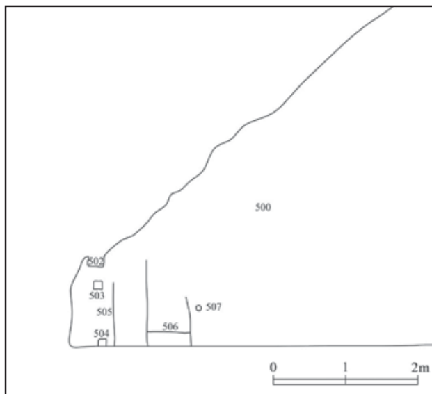
Fig. 14 - Ambiente H, prospetto F-F (S. D'Amico).
