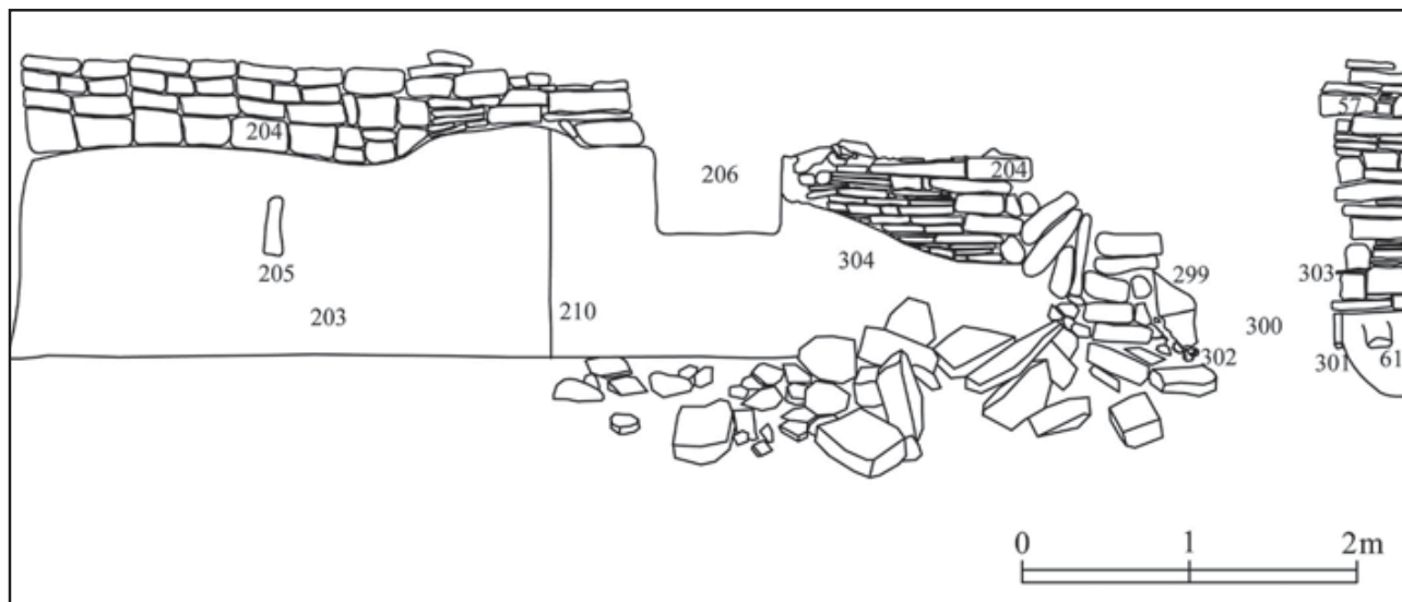
Fig. 5 - Ambiente C, prospetto A-A (S. D'Amico).
