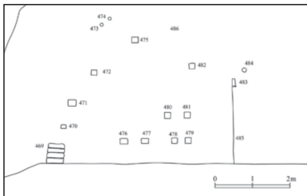
Fig. 12 - Ambiente E, prospetto D-D (S. D'Amico).
