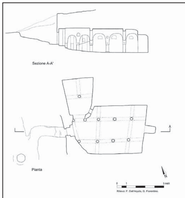
Fig. 7 - Il rilievo della moschea (grafica F. dell'Aquila e G. Fiorentino).
