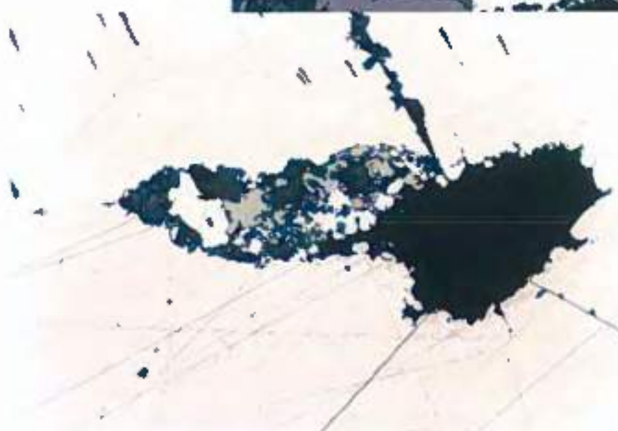
Foto 19: galena che racchiude una plaga con marcasite (bianca), tetrahedrite (grigia), anargite (rosata), covellina (azzurra) e carbonati (grigio-neri) (20X, N/I), miniera S. Patrizio (foto M.L. Perissinotto)
