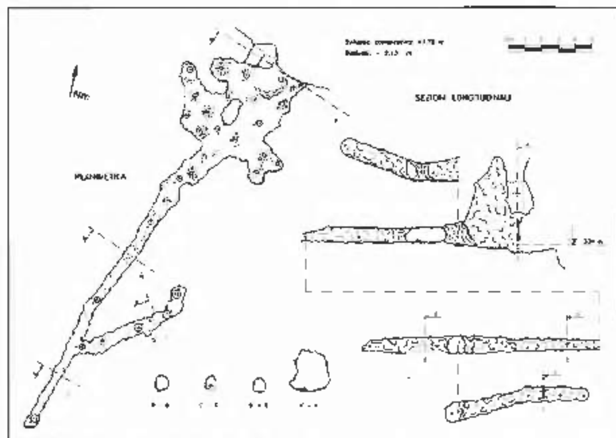
Fig. 19: planimetria e sezione longitudinale della miniera Orco D2. CA 99 V VI (Équipe Veneziana di Ricerca, rilievo L. Ferioldi, F. Maglich, M. L. Perissinotto - 2001; grafica I. Ferrakli - 2001)
