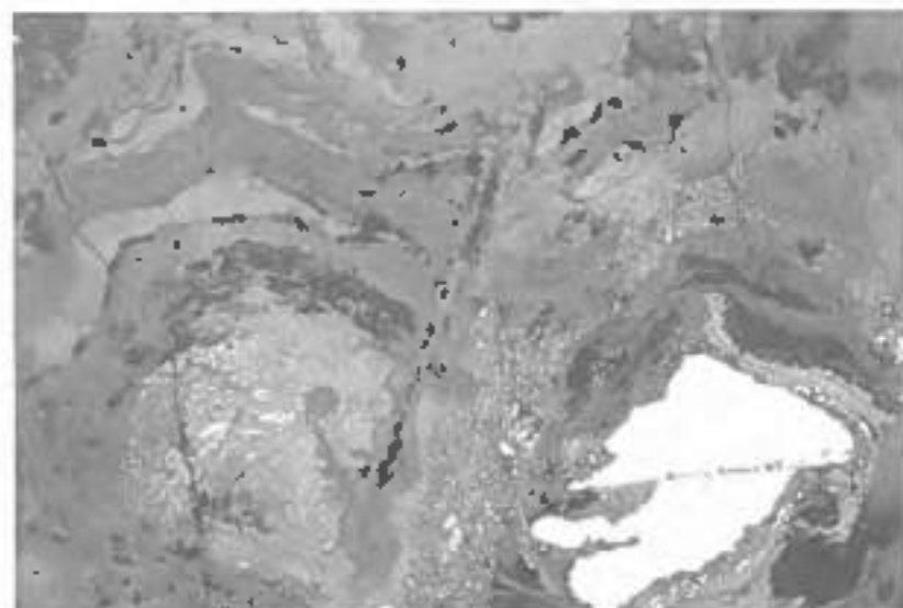
Foto 20: galena (bianca) fratturata ed estesamente alterata in cerussite e anglesite. Nelle croste di alterazione è precipitata della galena secondaria finemente polverizzata (6x, 14/1), miniera Busi 01 (foto M.L. Perissinotto).
