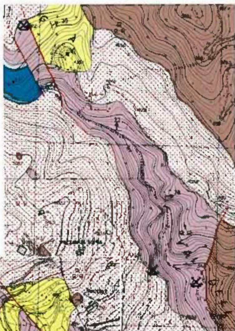
Fig. 8: assetto geologico della zona della valle dell'Orco e ubicazione delle miniere argentifere studiate (da Perissinotto, 1999, modificata). Legenda a pagina seguente
