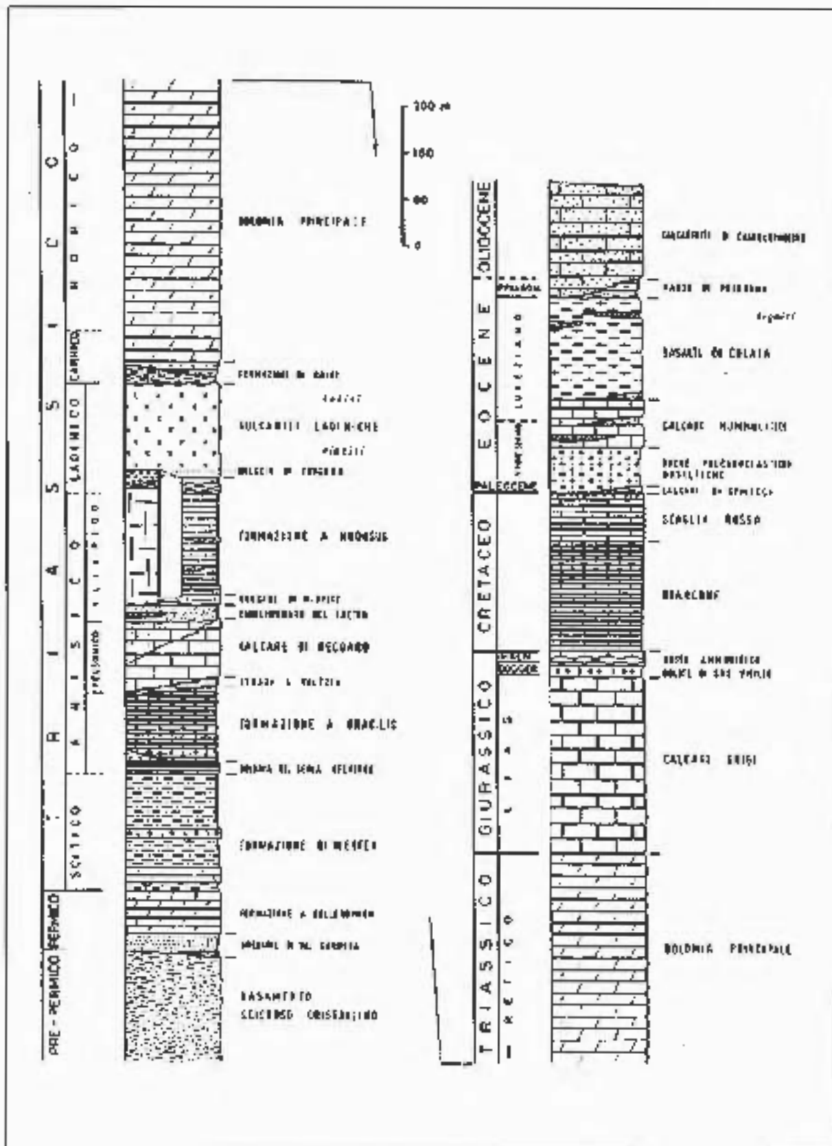
Fig. 6: successione stratigrafica schematica del Recoarese (da Barbieri et al. , 1980).
