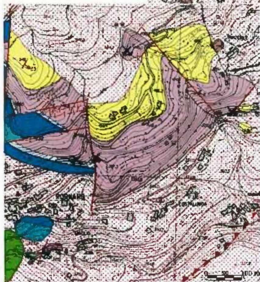
Fig. 9: assetto geologico della zona di Pomaio - Pozzani e ubicazione delle miniere argentifere studiate (da Perissinotto, 1999, modificata). Legenda a pag. seguente.
