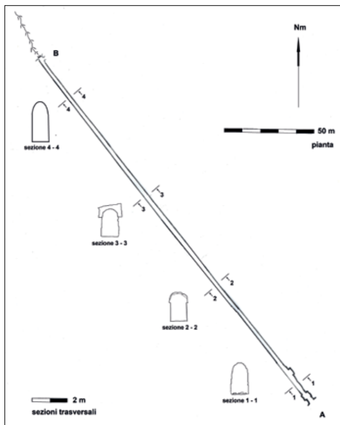
Fig. 13 – Pianta del rilievo dell'Emissario del Pantano. A: ingresso Emissario del Pantano; B: uscita Fontana fredda (topografia di A. Pedicone Cioffi, N. Sbordonì, M. Parente, M. Mugione, G. Masiello, V. Poole; elaborazione grafica S. Gambari).
