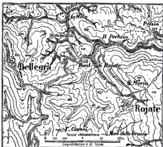
FRASO DI SITUAZIONE DELLA GROTTA DELL'ARCO DI BELLEGRA (C. 3 - La)
